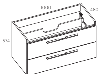
ТУМБА ПОД УМЫВАЛЬНИК 100 NSS
