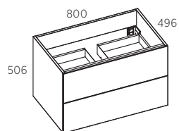
ТУМБА ПОД УМЫВАЛЬНИК 80
