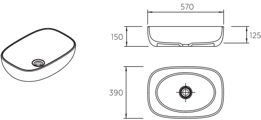
РАКОВИНА НА СТОЛЕШНИЦЫ
