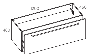
ТУМБА ПОД УМЫВАЛЬНИК 120 (2 ящика)
