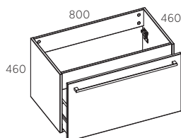
ТУМБА ПОД УМЫВАЛЬНИК 80 (2 ящика)
