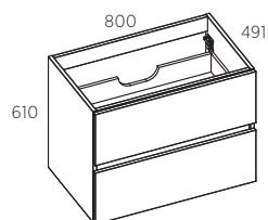
ТУМБА ПОД УМЫВАЛЬНИК 80
